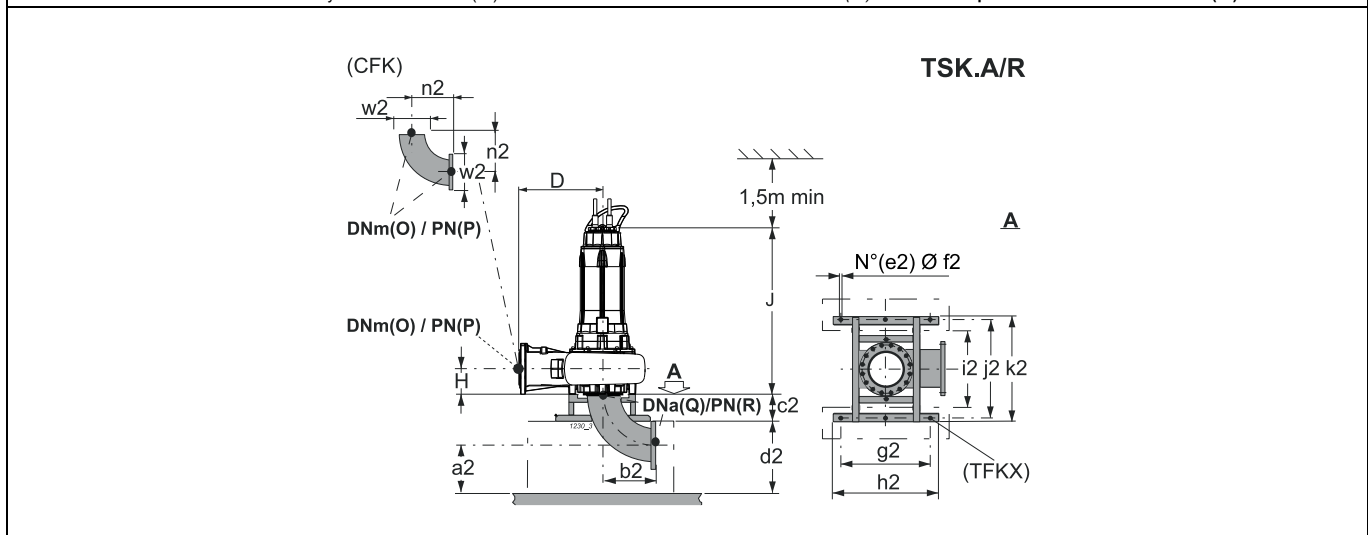
For fixed installation in a dry chamber - vertical (R) / Pour installation fixe en fosse sèche - verticale (R) / Esecuzione per camera asciutta - verticale (R)
